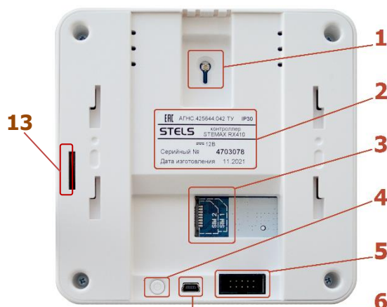
Рисунок А.2 — Основание корпуса контроллера
