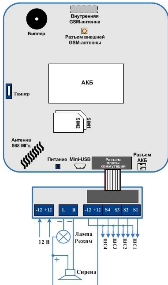
Рисунок А.6 — Схема внешних подключений контроллеров с ревизиями платы 1.0—1.2
