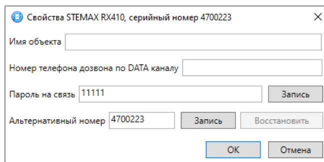
Рисунок 4.48 — Окно Свойства
