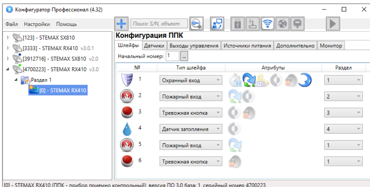
Рисунок 4.31 — Вкладка Шлейфы
