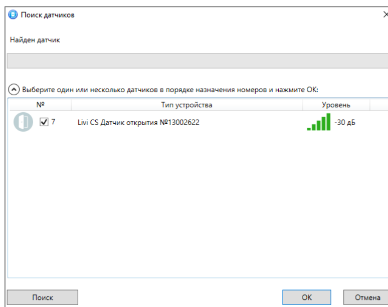
Рисунок 4.35 — Поиск радиоустройства
