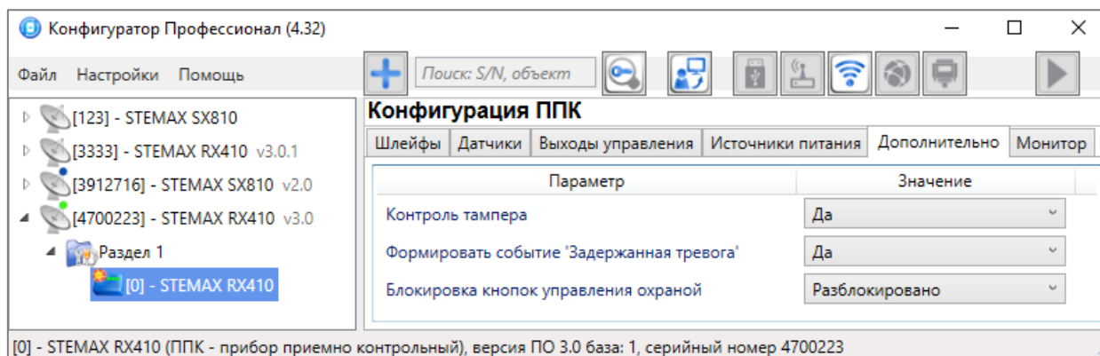
Рисунок 4.42 — Вкладка Дополнительно
