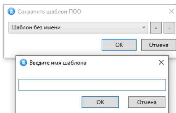
Рисунок 4.46 — Сохранение шаблона
