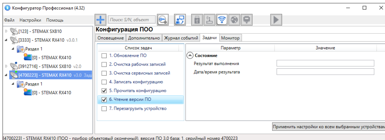
Рисунок 4.20 — Вкладка Задачи
