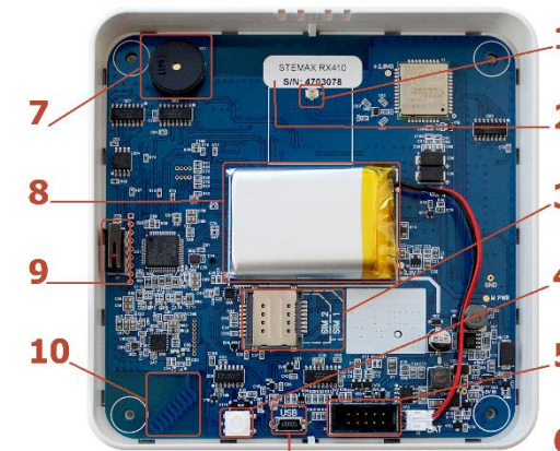
Рисунок А.3 — Плата контроллера (ревизия 1.0)
