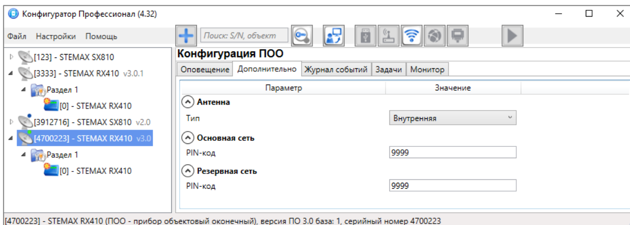
Рисунок 4.17 — Вкладка Дополнительно
