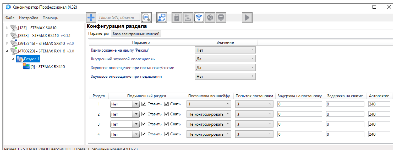
Рисунок 4.26 — Вкладка Параметры
