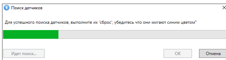
Рисунок 4.34 — Поиск радиоустройства
