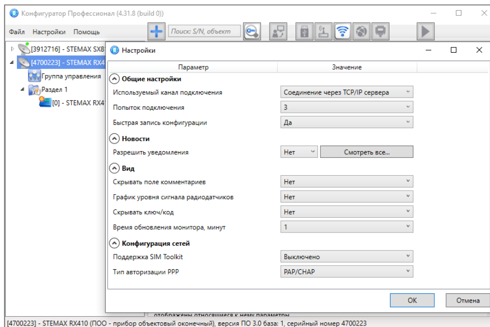
Рисунок 4.9 — Окно Настройки
