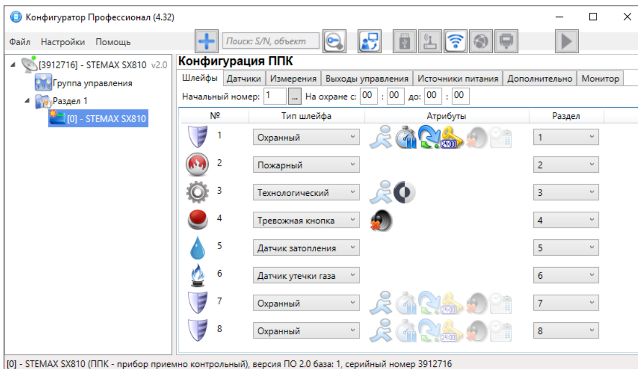
Рисунок 4.40 — Вкладка Шлейфы
