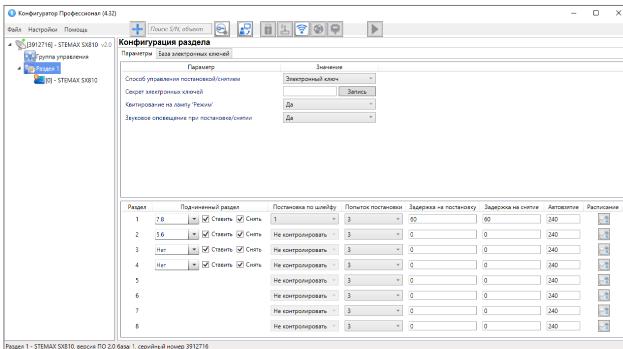
Рисунок 4.33 — Вкладка Параметры
