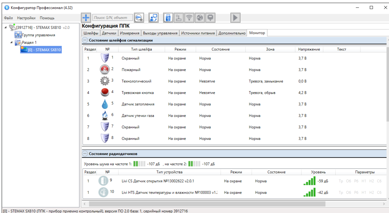
Рисунок 4.28 — Вкладка Монитор
