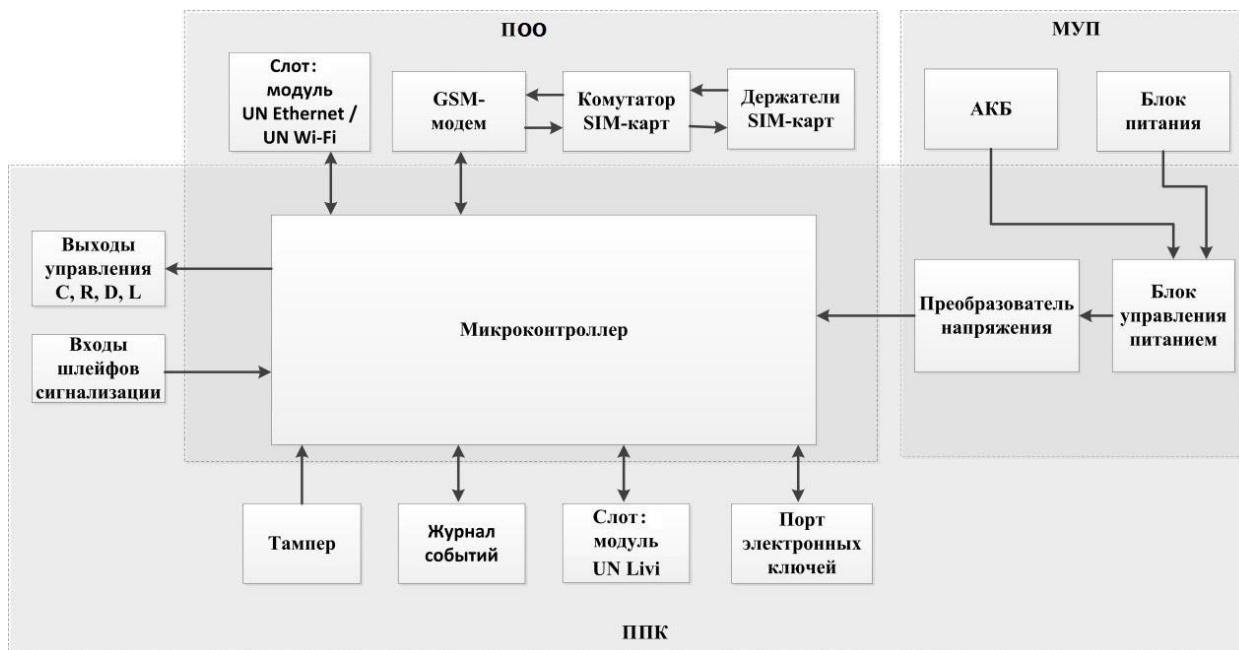
Рисунок 1.1 — Функциональная схема
