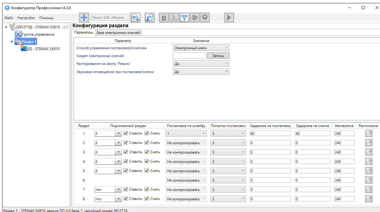
Рисунок 4.35 — Пример 1
