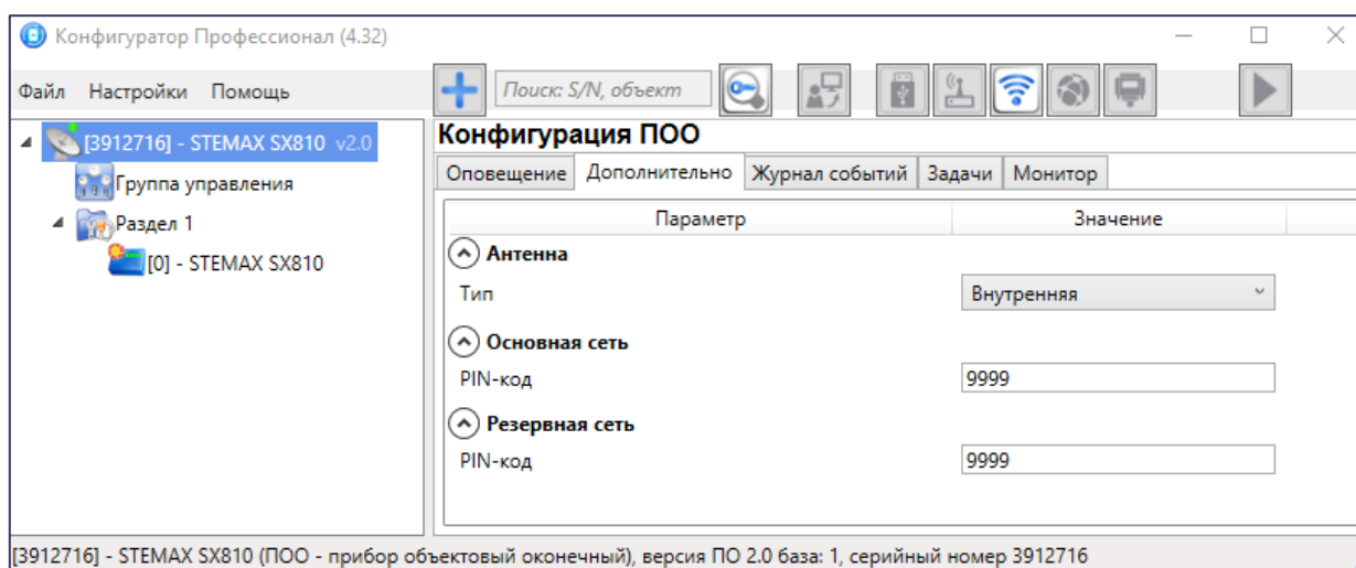
Рисунок 4.24 — Вкладка Дополнительно
