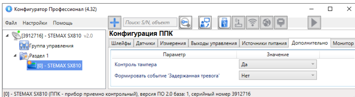
Рисунок 4.51 — Вкладка Дополнительно
