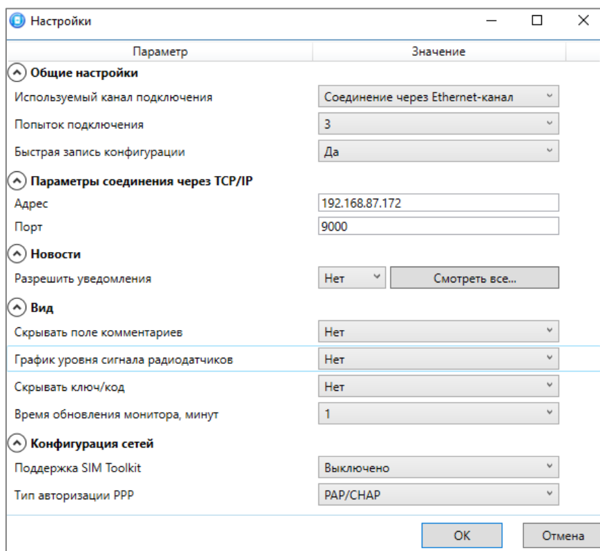
Рисунок 4.11 — Окно Настройки
