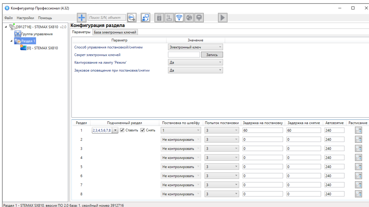
Рисунок 4.36 — Пример 2
