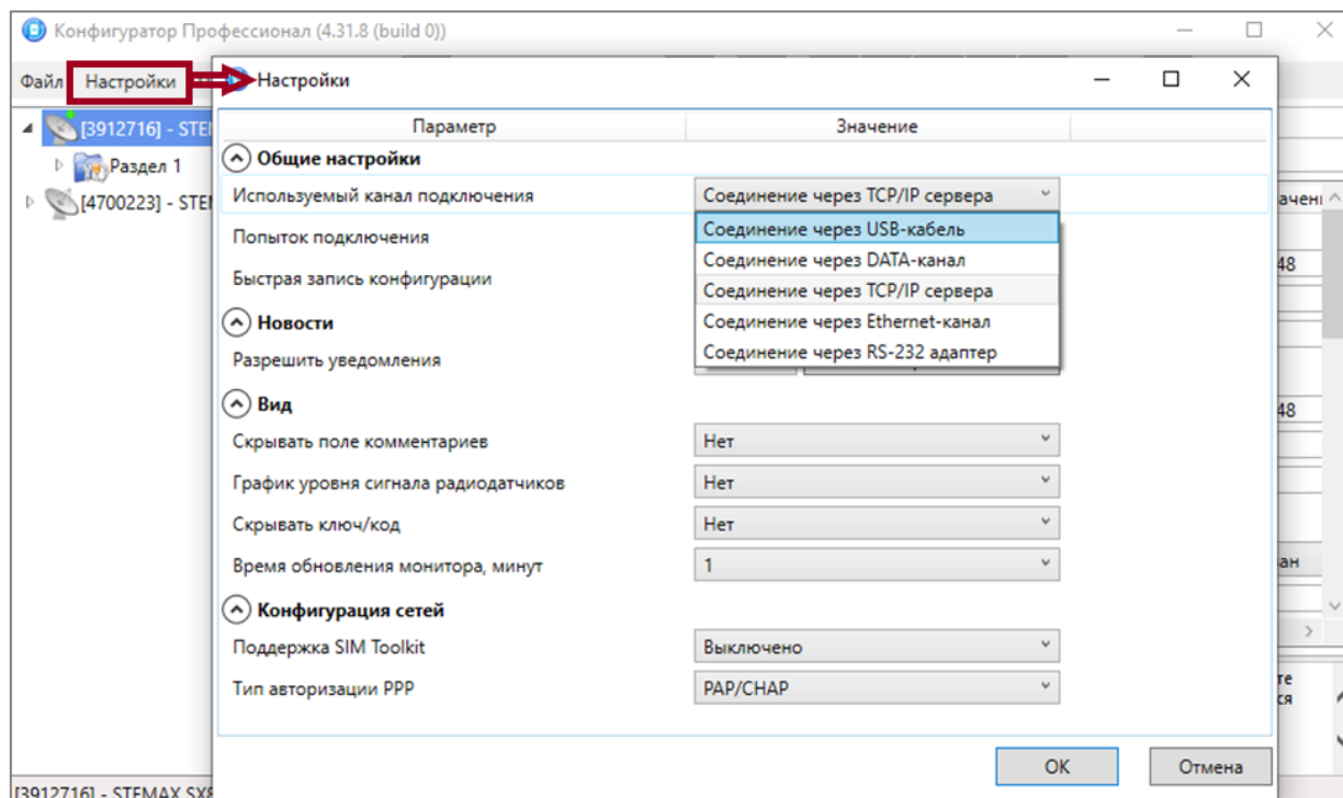
Рисунок 4.9 — Окно Настройки
