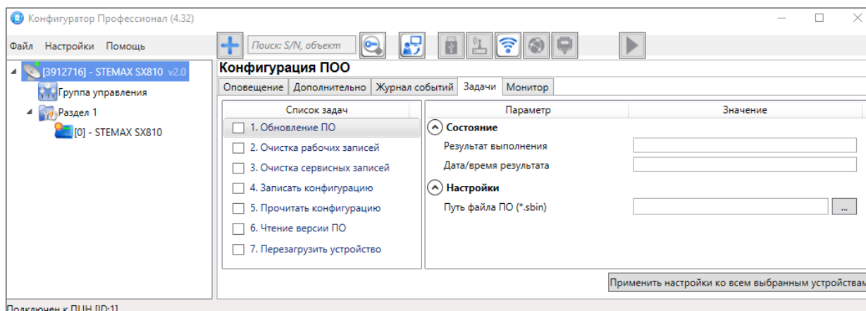
Рисунок 4.27 — Вкладка Задачи
